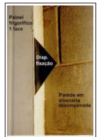
Detalhe da fixação painel 1 face para Adega climatizada personalizada
