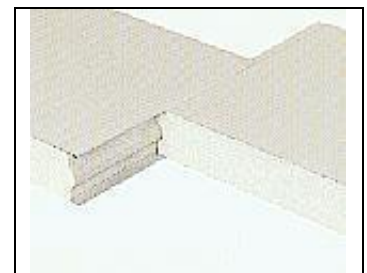
Detalhe do encaixe painel 2 faces para Adega climatizada personalizada
